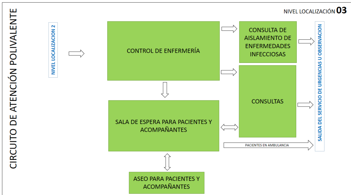
Figura 10. Diagrama de relaciones del Nivel de Localización 3 del Servicio de Urgencias de Hospitales. Circuito de Atención Polivalente.
