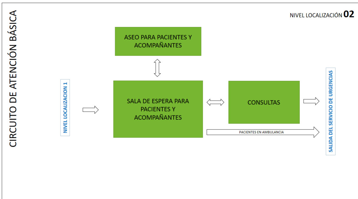
Figura 7. Diagrama de relaciones del Nivel de Localización 2 del Servicio de Urgencias de Hospitales. Área de Consultas: Circuito de Atención Básica.
