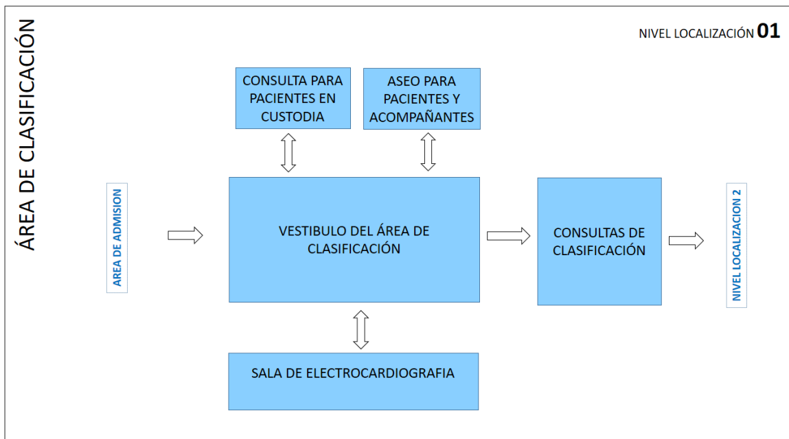
Figura 5. Diagrama de relaciones del Nivel de Localización 1 del Servicio de Urgencias de Hospitales. Área de Clasificación.
