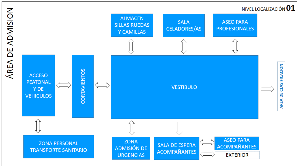
Figura 4. Diagrama de relaciones del Nivel de Localización 1 del Servicio de Urgencias de Hospitales. Área de Admisión.
